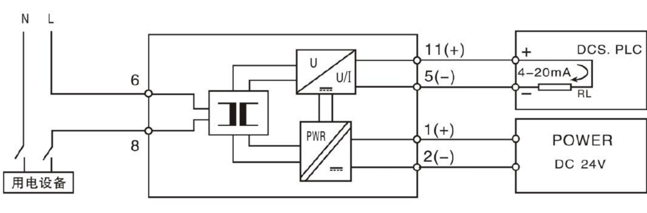
一进一出（DC 24V供电）
